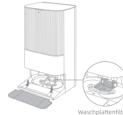
Waschplattenfilter
